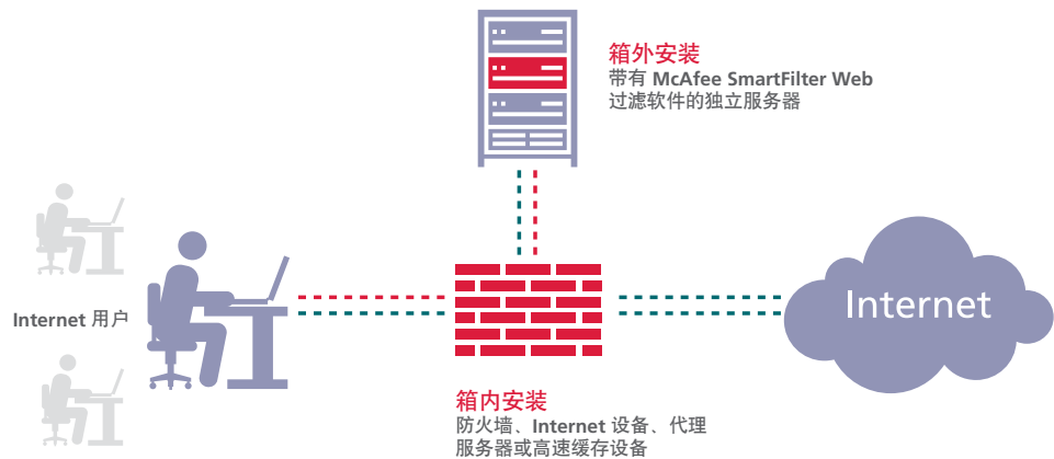
此图表示 McAfee SmartFilter 产品的典型配置。也可能为其他配置。
